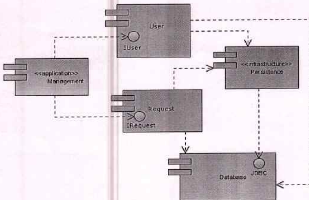
Fig: 2.4.7. Component diagram.
